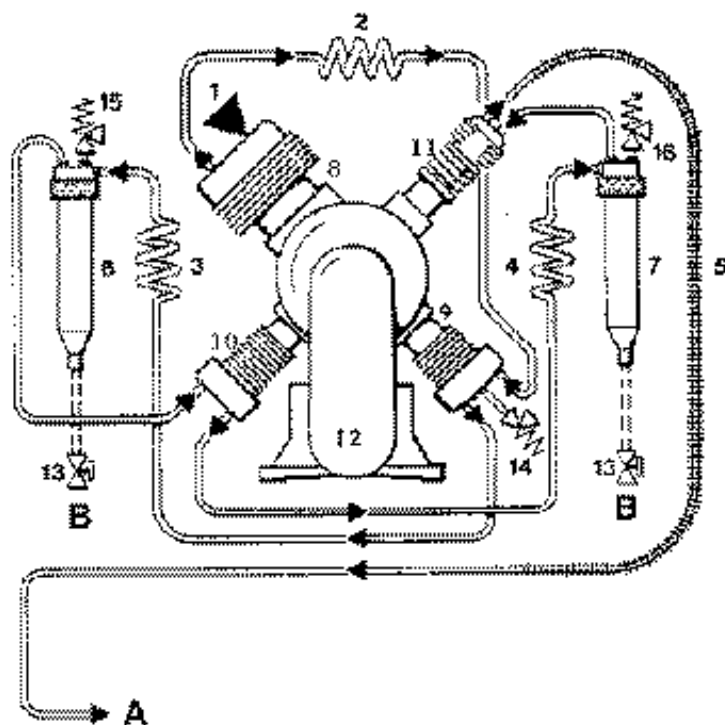
SHEMA VISOKOTLAČNEGA KOMPRESORJA:
